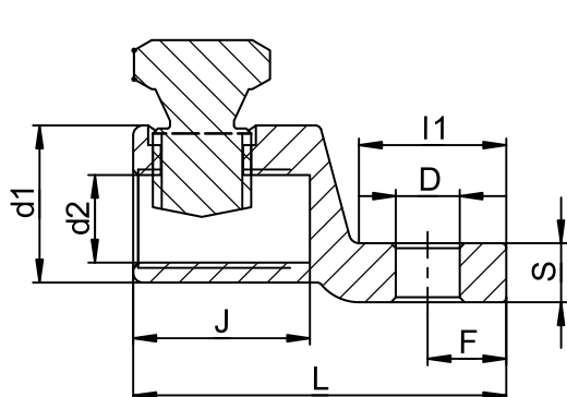
Чертеж наконечника 1НБ
