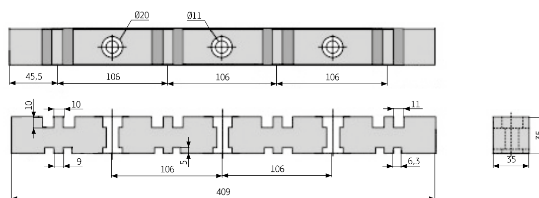
ИШП 4Р 409 мм
