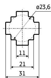
TT-B100
