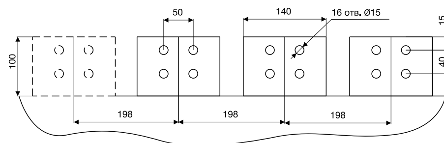
Силовые выводы E5K-3L
