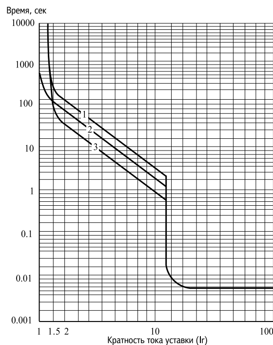
АПД-03 0,16-32 А
