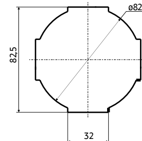
TT-B80
