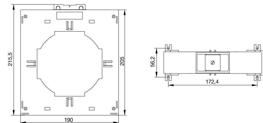
TT-B120
