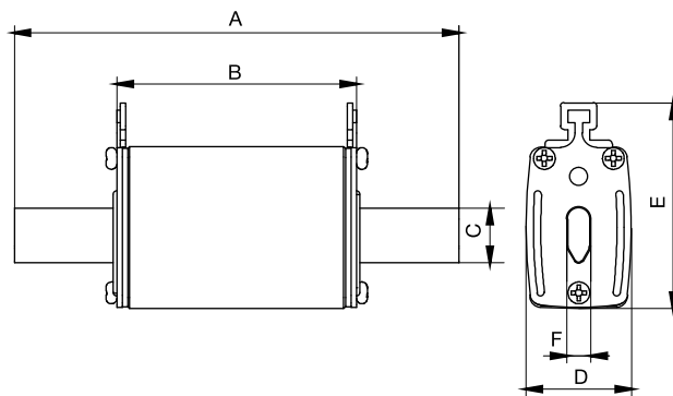
ППН-39
