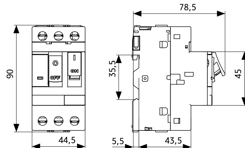
АПД-03 0,16-32 А
