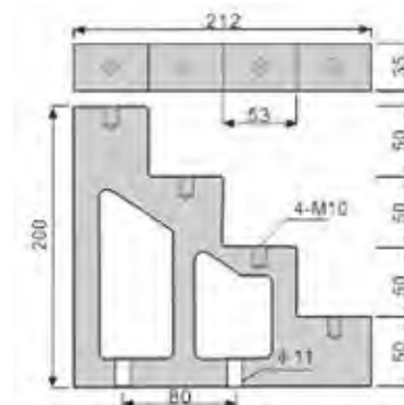
ИС4-50
