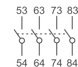
ПКЛ-40
