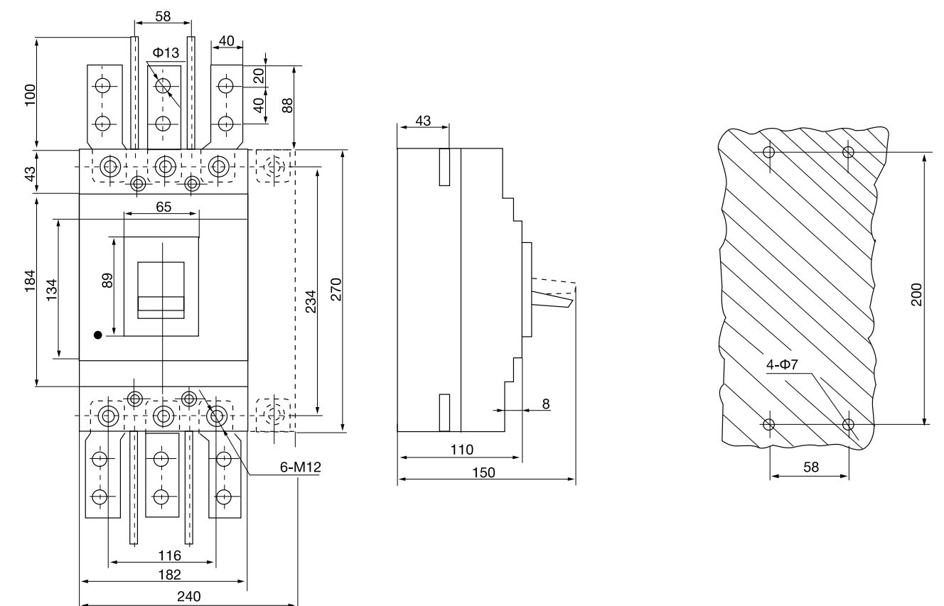
BA88-39
