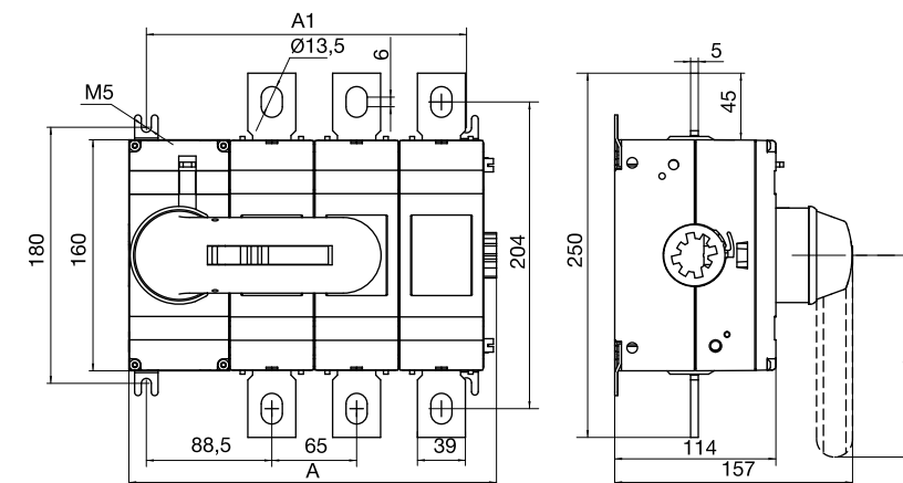
БНК-3933
