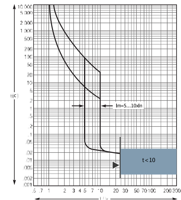
Термамагнитные расцепители TMR, 200-250 A
