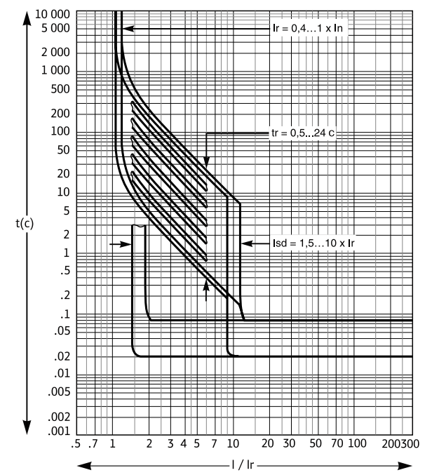
Электронный расцепитель ER3, 800-1600 A
