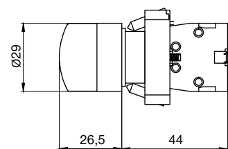
Стандартная черная
