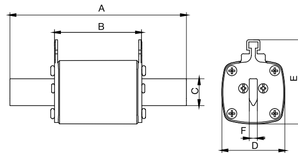
ППН-41
