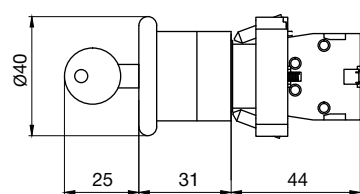
Грибок «СТОП» с ключом
