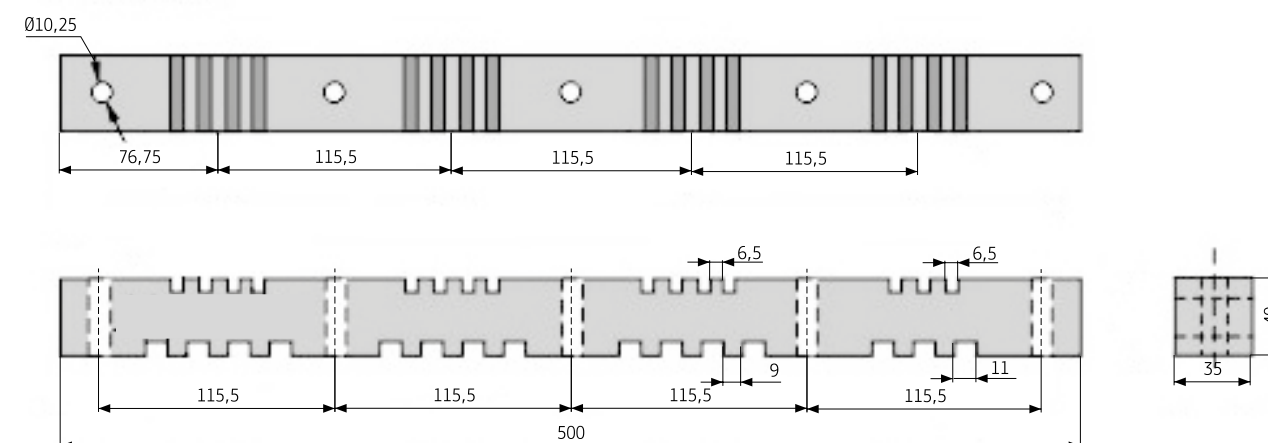
ИШП 4Р 500 мм
