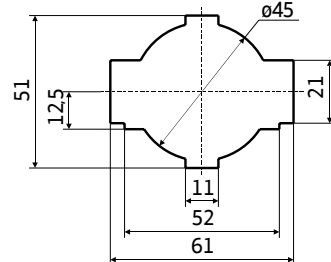
TT-B120
