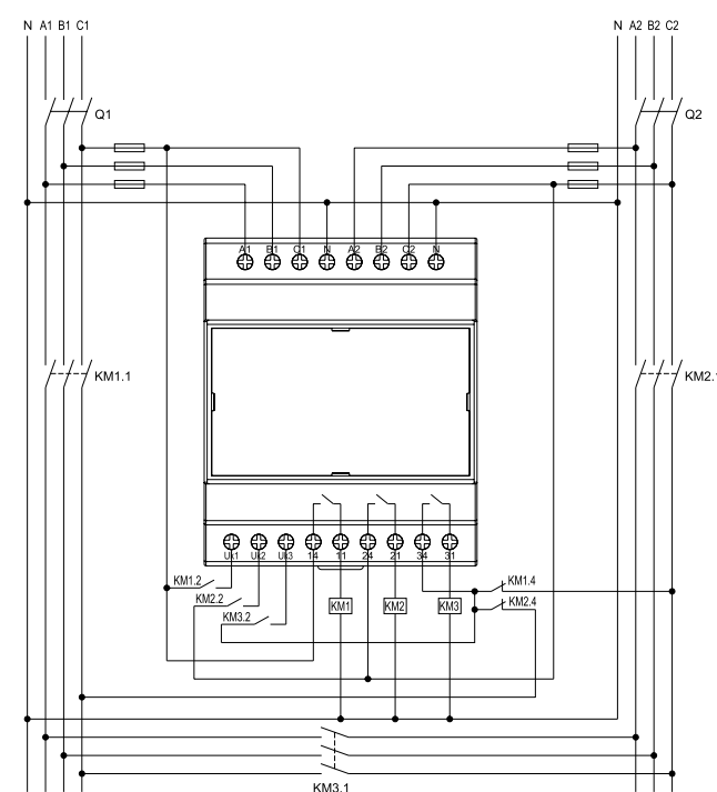
ETS-3ZC
