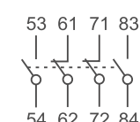
ПКЛ-22
