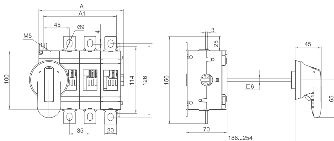
БНК-3534
