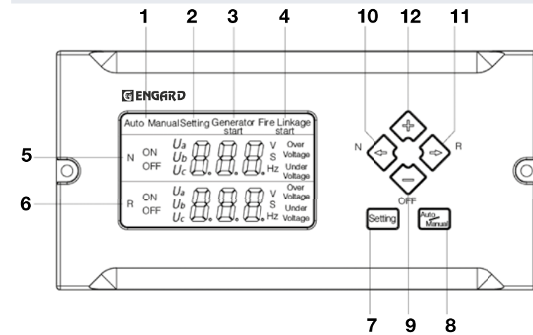
Панель универсального контроллера с ЖК-дисплеем
