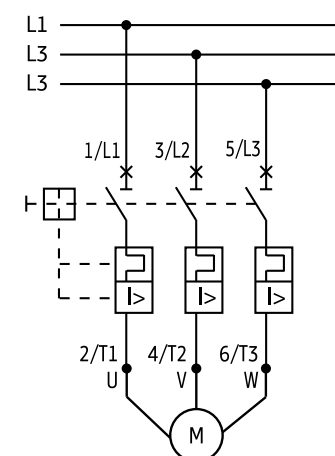
Подключение трехфазного двигателя
