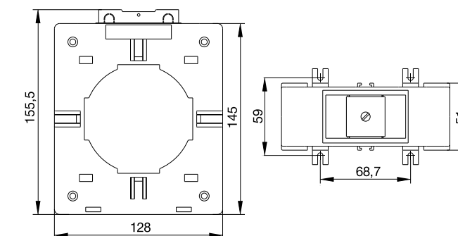
TT-B120
