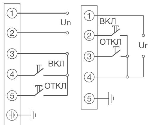
ED2KR-3/6
