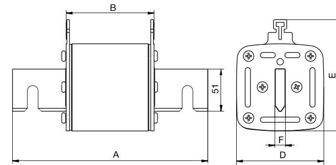
ППН-41
