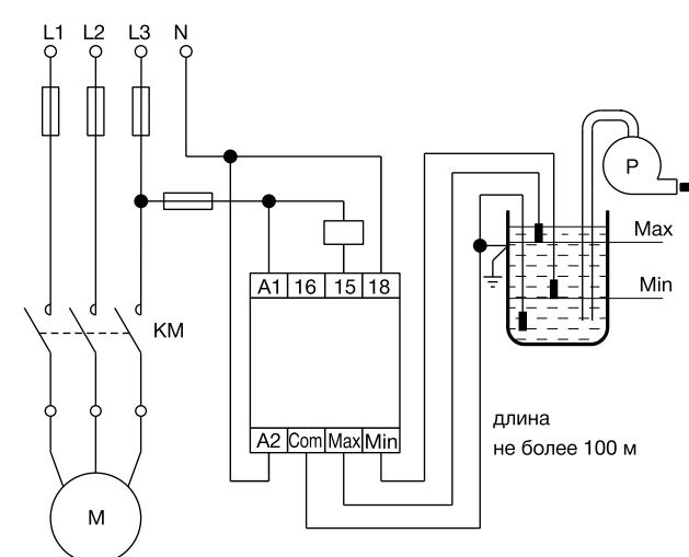
Откачивание жидкости из резервуара
