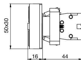
Двойная «ПУСК-СТОП»
