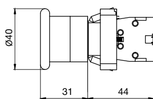
Грибок «СТОП»
