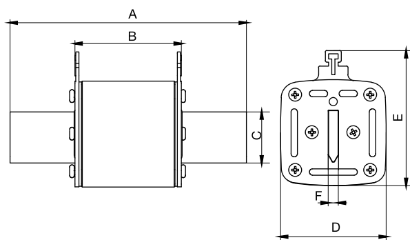
ППН-39
