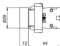
Плоская
