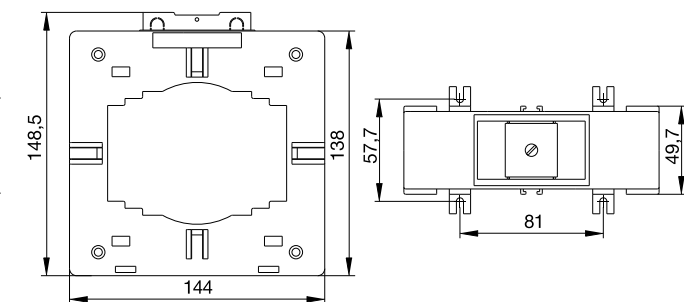
TT-B100
