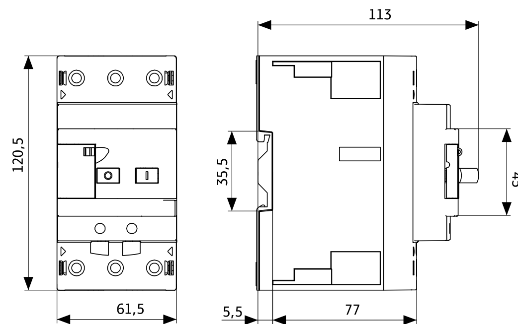
АПД-08 25-80 А
